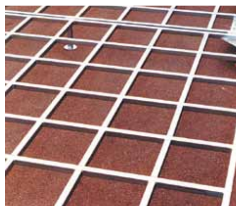
art. 3630 Piattaforma di sostegno zona caduta zincata a caldo con terminali gomma antiscivolo al mq Galvanised platform for high jump landing areas per sm
